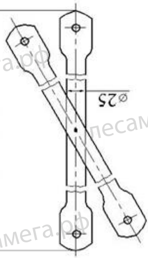
Диагональная связь (4)
