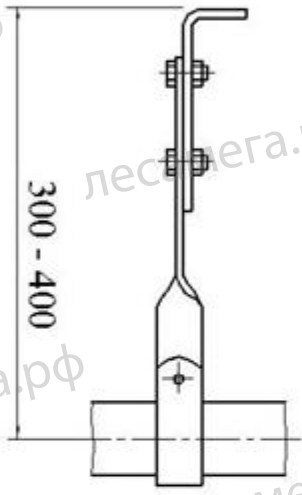
Кронштейн крепления (6)
