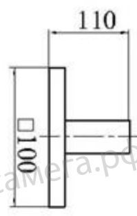
Опорная пятка (5)
